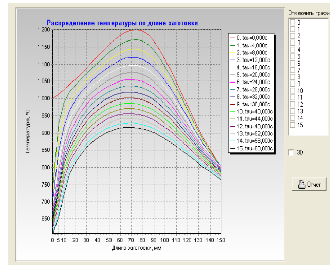
Рис. 2. Результаты моделирования распределения температур по высоте заготовки через различные промежутки времени ( \tau = \text{tau} ) от начала контакта заготовки и осадочной плиты
